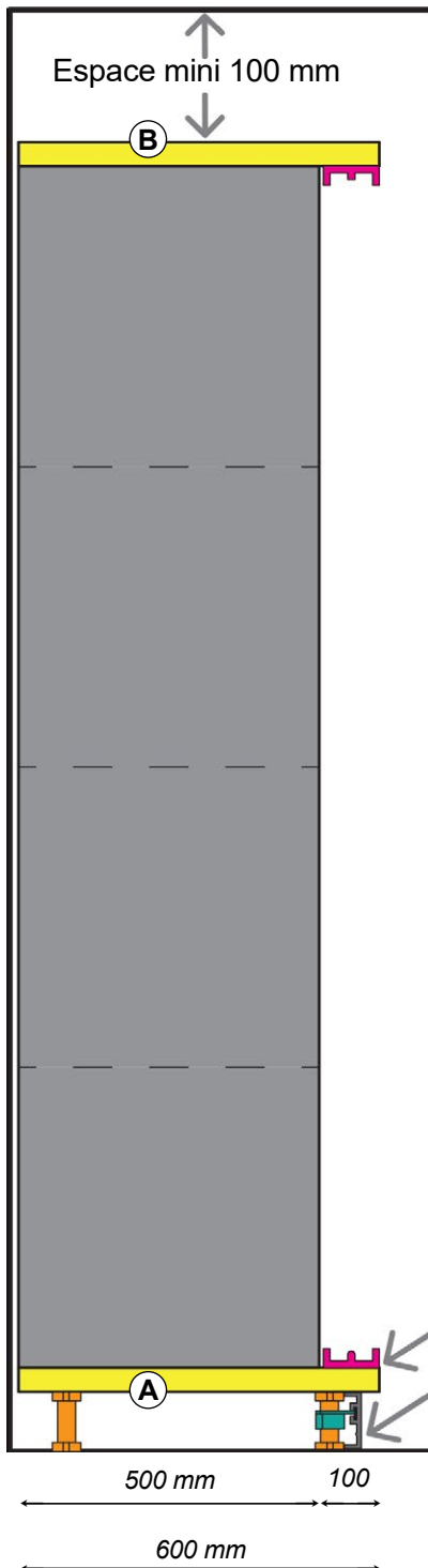
Vue latérale
